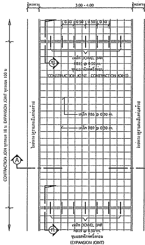
แปลนพื้นถนน
