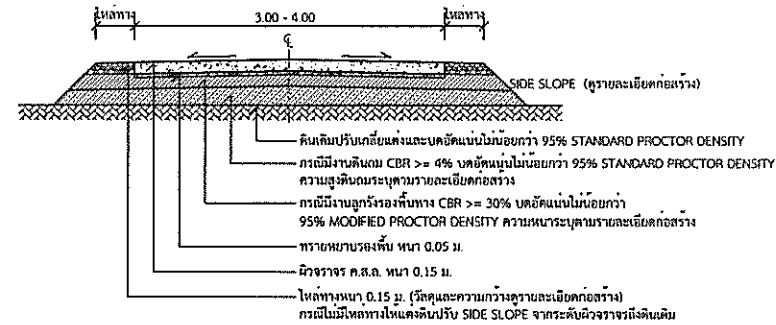
รูปตัด A-A 1 : 75
